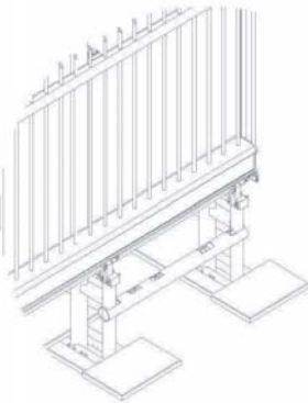
prefabfundering t.b.v. poortgeleiding en geleideportaal
