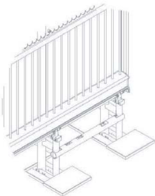
prefabfundering t.b.v. poortgeleiding en geleideportaal
